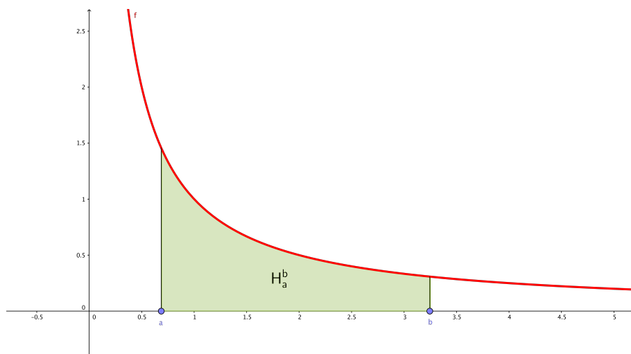
Figura 3: Hipérbole equilátera e área H_a^b
