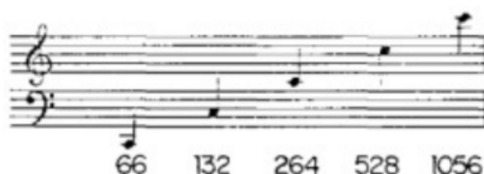
Figura 9: Notas musicais separadas em intervalos iguais correspondem a frequências em uma progressão geométrica
