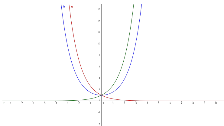
Figura 10: Gráfico de e^x , e^{-x} , e da catenária para a = 1
