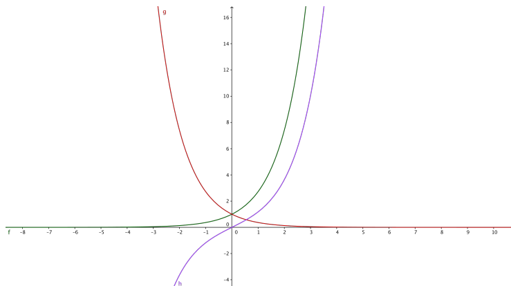
Figura 11: Gráfico de \frac{e^x - e^{-x}}{2}
